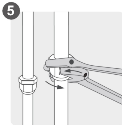
Kytke putkisto
