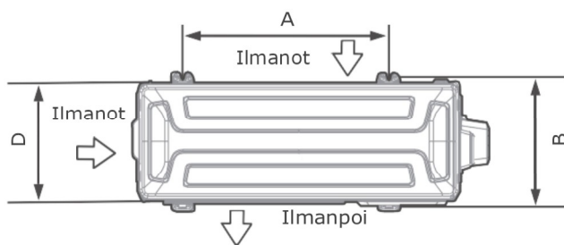
Yläkuva
