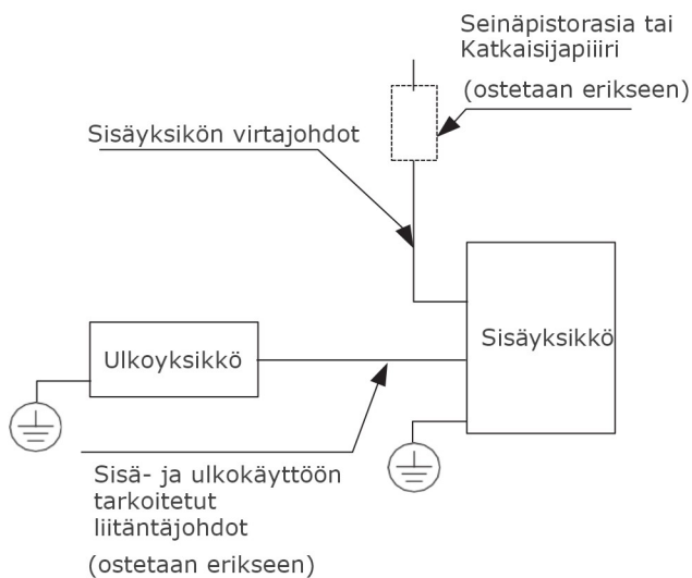
Sisätilojen virtalähdemallit
