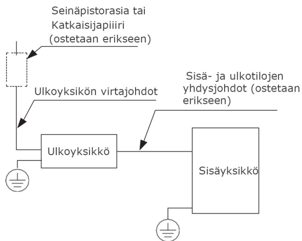
Ulkoilman virtalähdemallit
